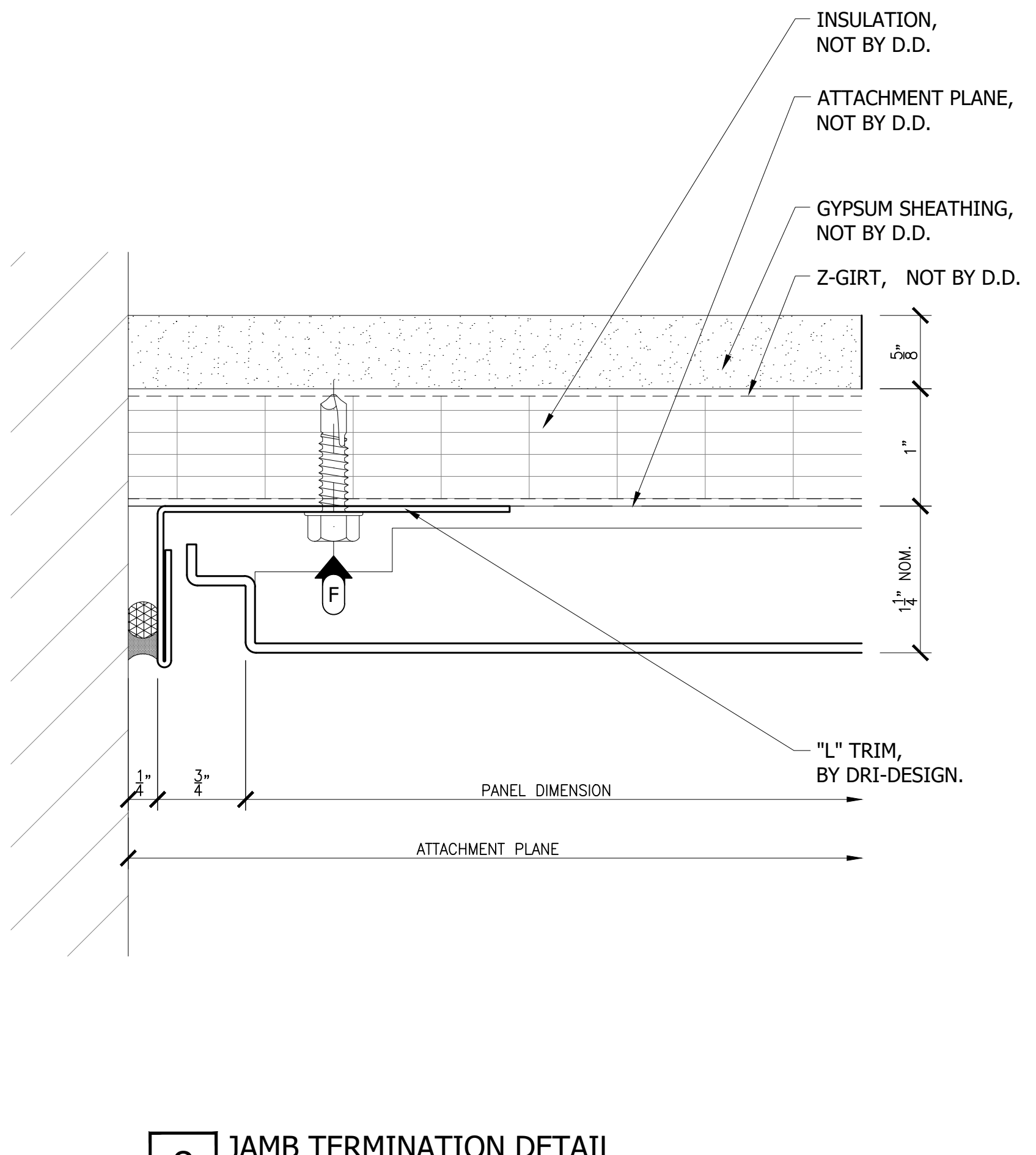
8 JAMB TERMINATION DETAIL REF: --/---
